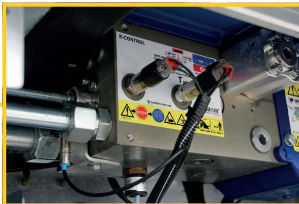
Oliedruk- en temperatuurvoersensor
